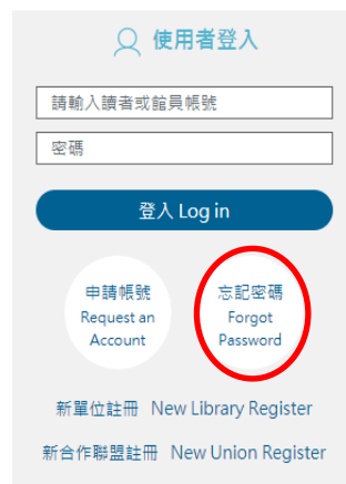
圖 2-9 登入 NDDS
